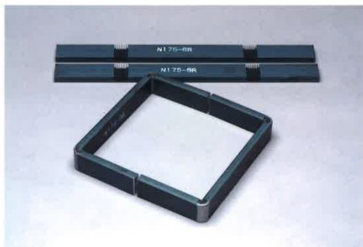
④スリット裏当金 (6mm専用裏当金)
